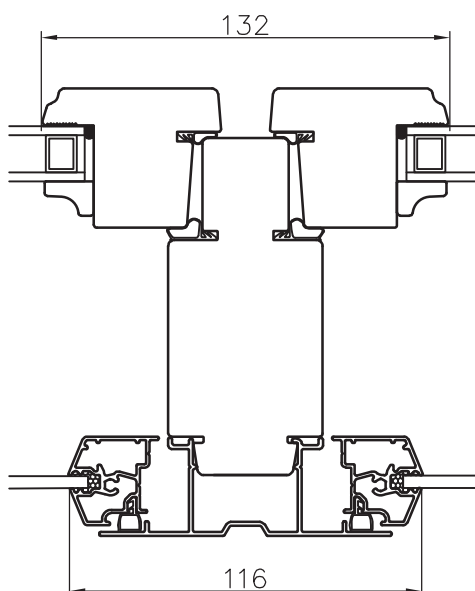
Vertikaalne impost
