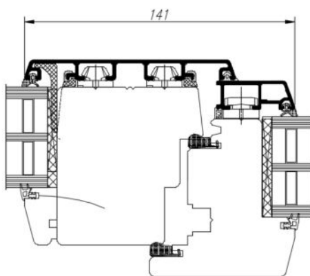
Vertikaalne impost
